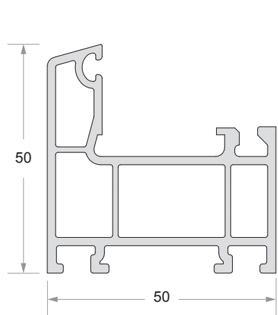
Casement Frame Code No : DP - 551
