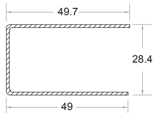
Door Sash Code No : ST - 556
