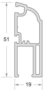
Mesh Sash Code No : DP - 510
