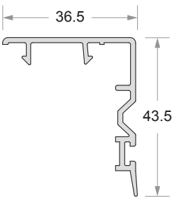
Door Interlock Code No : DP - 506
