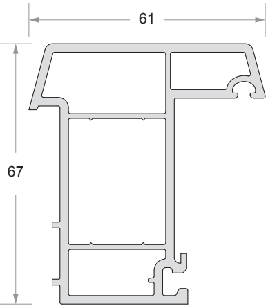
False Mullion Code No : DP - 757
