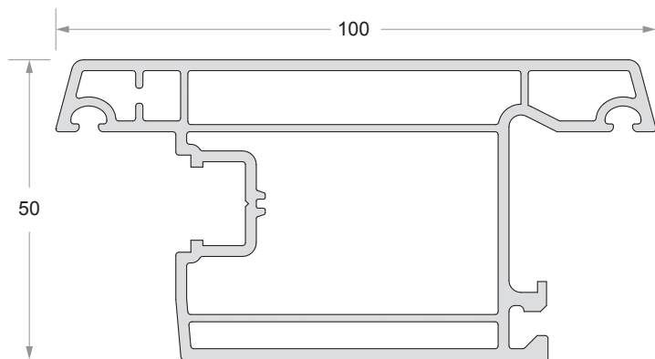
Door Sash Code No : DP - 556
