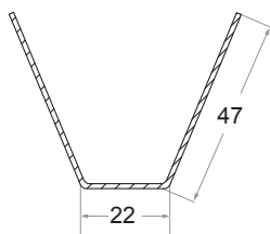
Corner Coupler 135° Code No : ST - 712
