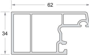
Sash / Style Code No : DP - 601
