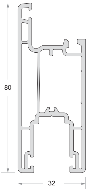
Sliding Door Sash Code No : DP - 504
