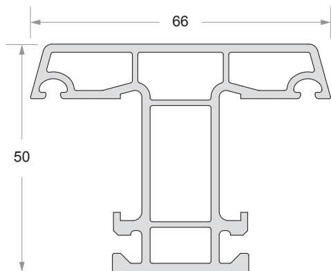
Sash / Mullion Code No : DP - 552
