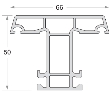
Sash / Mullion Code No : DP - 552
