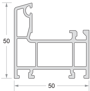
Casement Frame Code No : DP - 551
