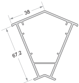
Corner Coupler 135° Code No : DP - 712
