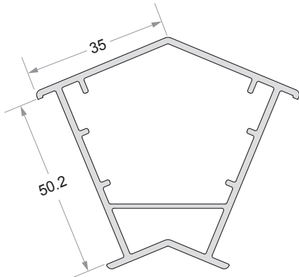
Corner Coupler Code No : DP - 512
