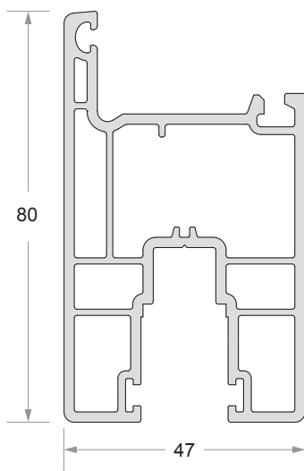
Sliding Door Sash Code No : DP - 704
