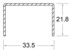
Door Sash Code No : ST - 704
