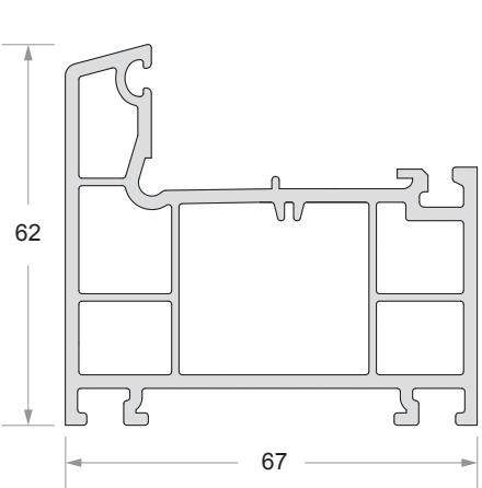
Casement Frame Code No : DP - 751
