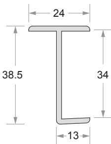
'T' Profile Code No : DP - 602
