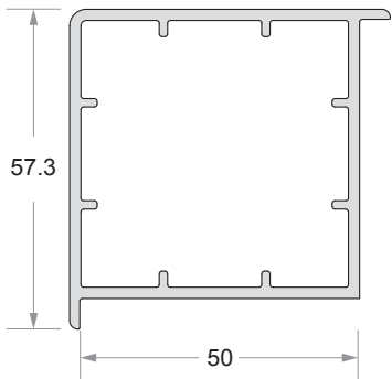
Corner Coupler Code No : DP - 511
