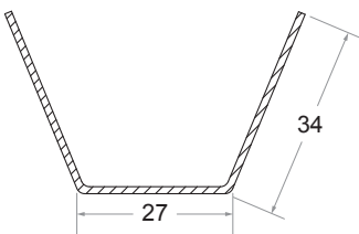
Corner Coupler 135° Code No : ST - 512
