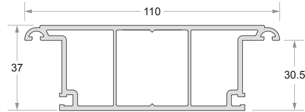
Door Mullion Code No : DPDS - 11037
