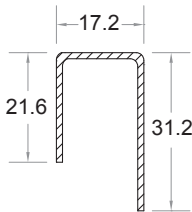
Door Sash Code No : ST - 504
