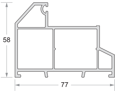
Door Frame Code No : DPDF - 7758
