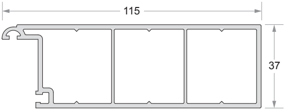
Door Sash Code No : DPDS - 11537
