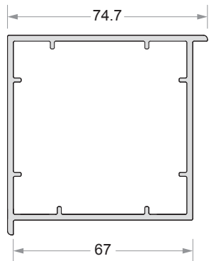
Corner Coupler 90° Code No : DP - 711
