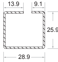
Casement Frame Code No : ST - 751
