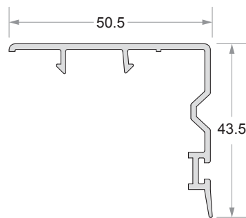
Door Interlock Code No : DP - 706
