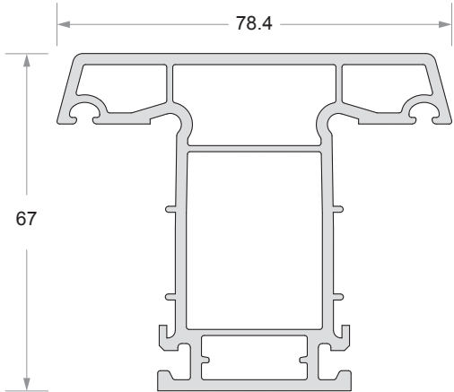
Sash / Mullion Code No : DP - 752
