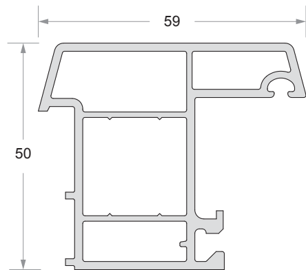
False Mullion Code No : DP - 557
