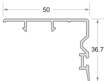
Window Interlock Code No : DP - 705
